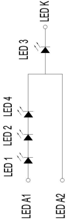
BLU circuit
